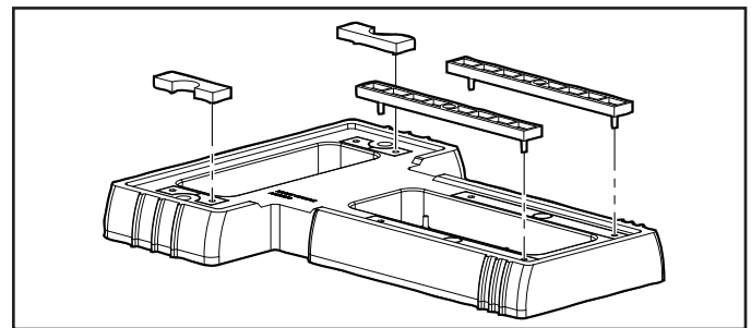
Figure 7. Enclencher les entretoises en place
