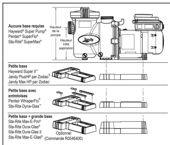
Figure 5. Configurations de base (modèle VS FloPro uniquement)
