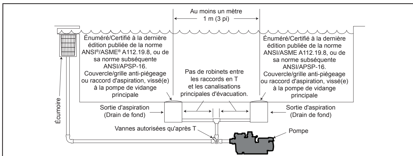
Figure 4. Nombre de prises d'aspiration par pompe
