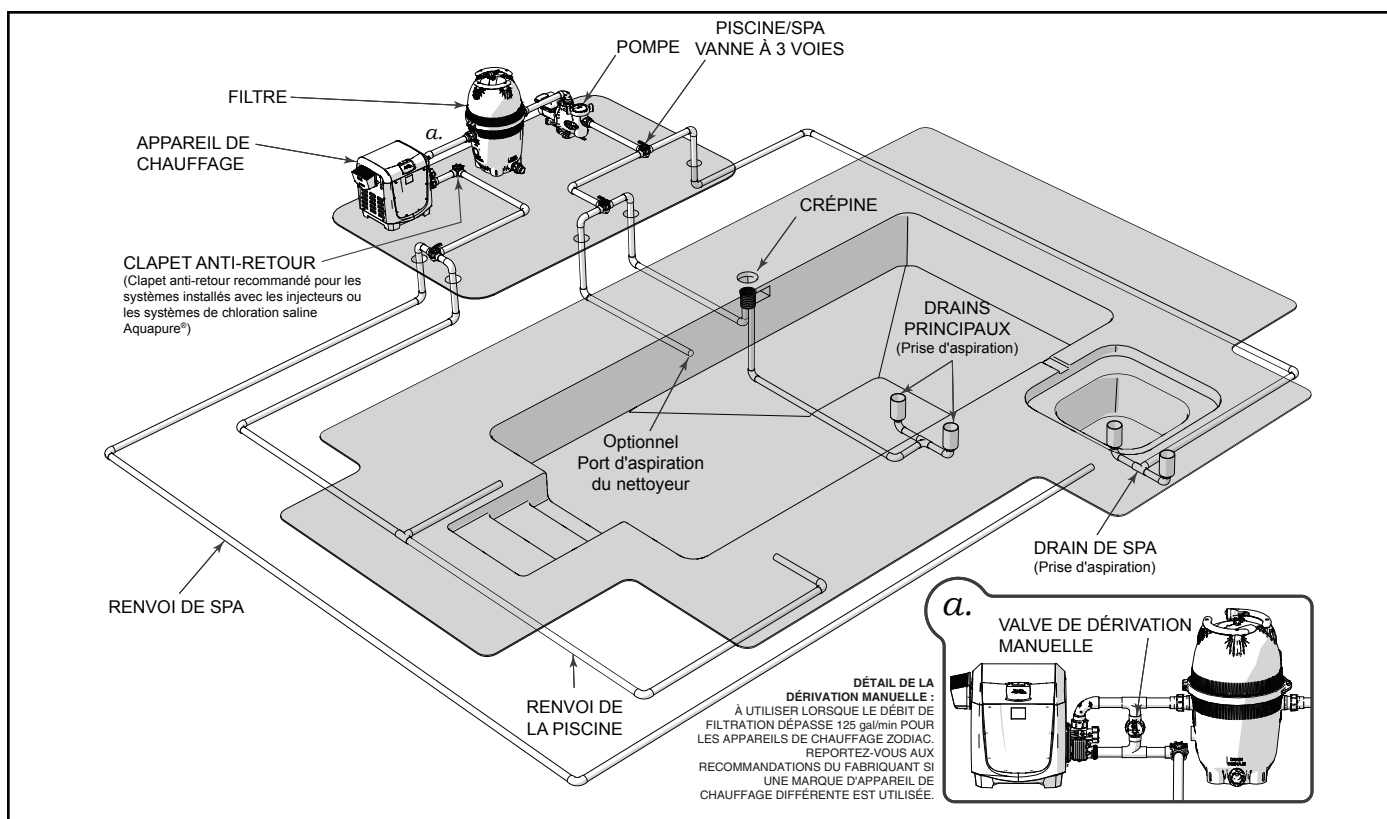
Figure 3. Installation de la tuyauterie typique
