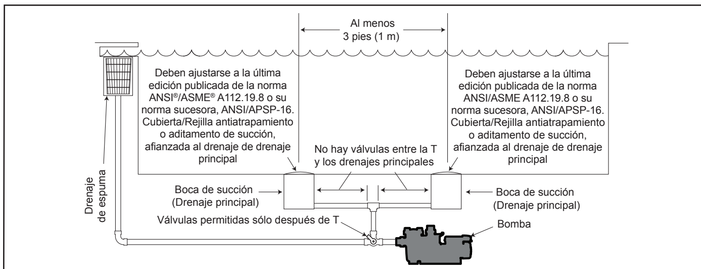
Figura 4. Cantidad de salidas de succión por bomba
