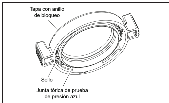
Figura 11. Junta tórica de prueba de presión azul
