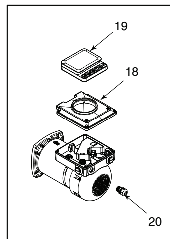
Vista ampliada del motor/accionador (Modelos de bomba que terminan en DVS)
