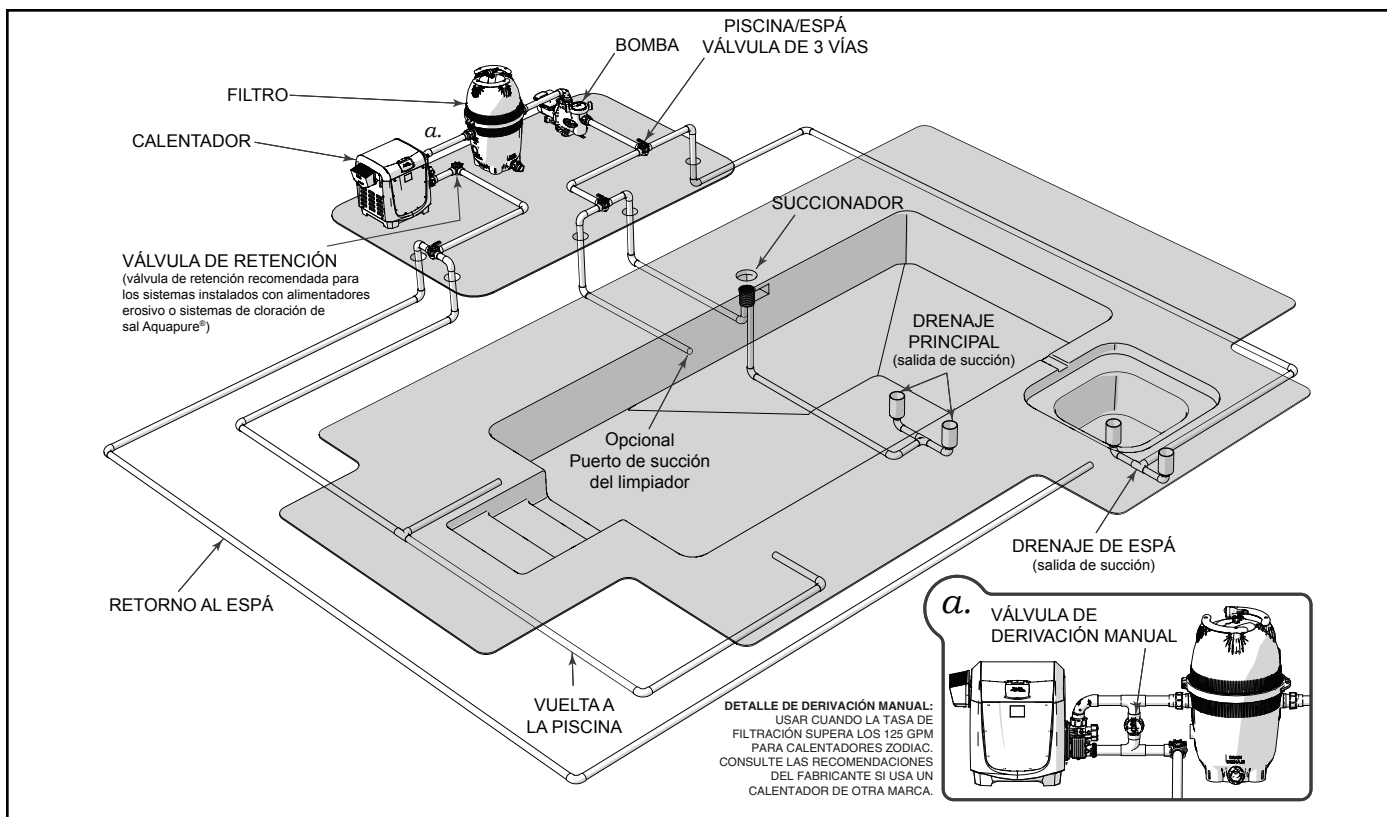
Figura 3. Instalación típica de las tuberías
