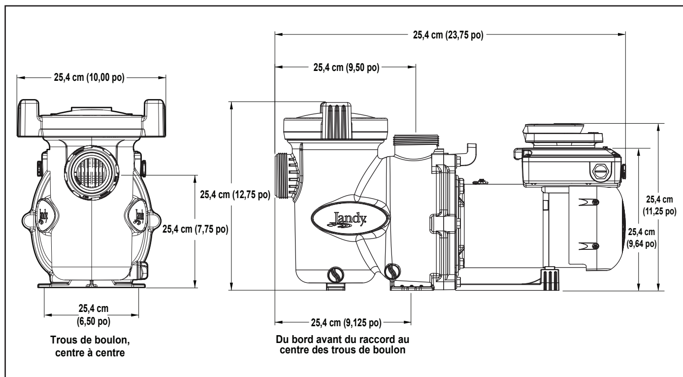
Figure 1. Dimensions de la Pompe à vitesse variable
